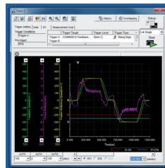
Anzeige der SERVOPACK-Daten auf einem Computer wie auf einem Oszilloskop
